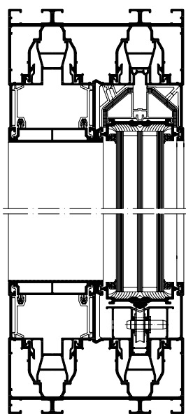
Κατακόρυφη τομή, Κλίμακα 1:6 Vertical unit section detail, Scale 1:6
